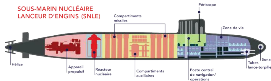
Vue en coupe d'un sous-marin nucléaire lanceur d'engins (SNLE) de classe Le Triomphant, outil principal de la dissuasion nucléaire française.
